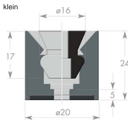
Art. Nr. | Abmessungen SI9-KOMPL. | siehe Zeichnung
