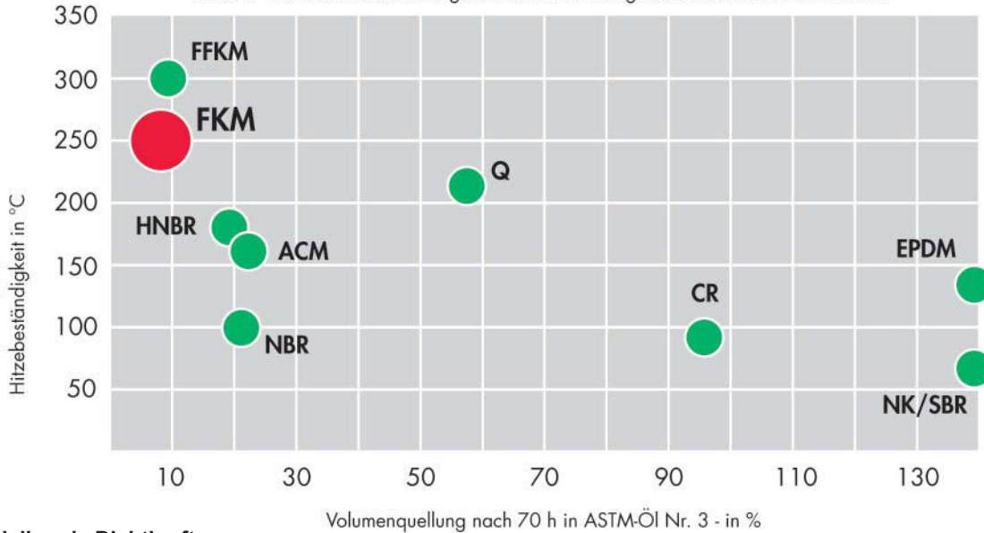
Abb. 3 - Hitze und Ölbeständigkeit von FKM im Vergleich mit anderen Elastomeren
