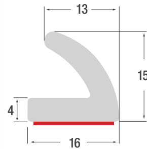
Fahnenprofil E1524D-AF in schwarz EPDM
