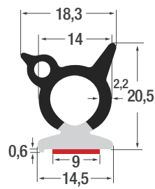
Sonderprofil 8656/00-M-T-01 EPDM Weich-Moosgummi
