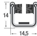
830 R Fensterführung für Glasstärke 6 mm EPDM beflokt
