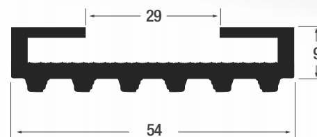
Schutzprofil P071 in schwarz EPDM
