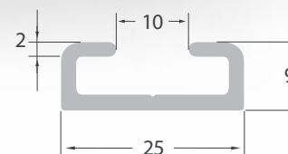
Aluprofil 080111 für Gummidichtung
