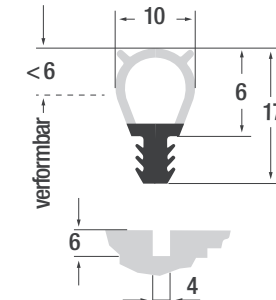
Steckprofil P209 - 0704 EPDM Weich-Moosgummi
