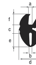
Gummi-Klemmprofile in schwarz EPDM
