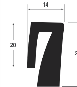
Sonderprofil P710 in schwarz EPDM 45° Shore
