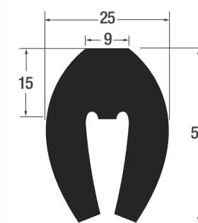
Schutzprofil U9/15 in schwarz EPDM 60° Shore
