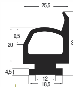
Schutzprofil P080 in schwarz EPDM
