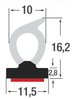
Sonderprofil 8637/00-MT EPDM Weich-Moosgummi
