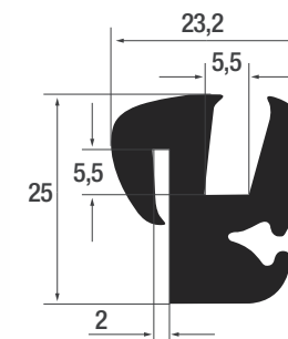
Verglasungsprofil U9/15 in schwarz EPDM 60° Shore
