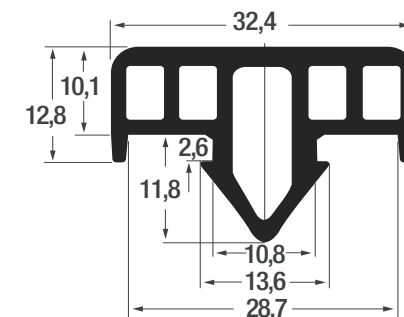
Glasauflageprofil P004/PVC/K in schwarz PVC
