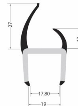
Fahrzeugaufbautendichtung P200701 in schwarz/weiß PVC - weich / PVC - hart
