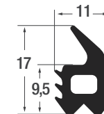
Zargenprofil P020001 in schwarz PVC-weich
