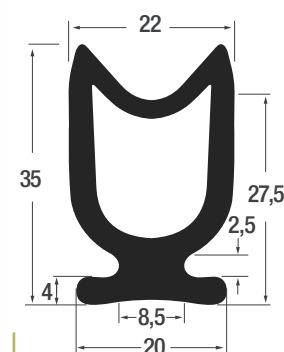
Fingerschutzprofil P142 in schwarz EPDM
