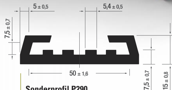
Sonderprofil P290 in schwarz EPDM
