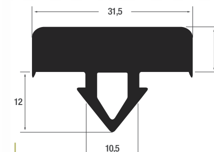
Glasauflageprofil P004/GI/Voll in schwarz EPDM
