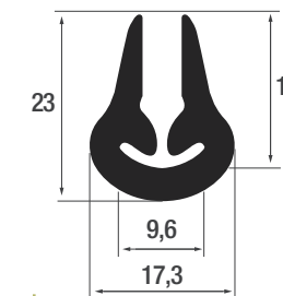
Sonderprofil P002 in schwarz EPDM
