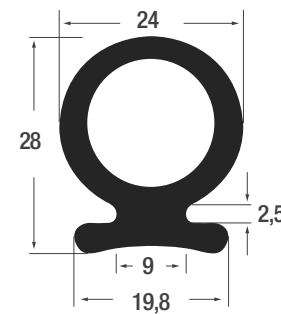
Sonderprofil P02A069 in schwarz EPDM
