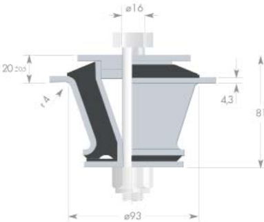
Art. Nr. 786026S3 NK 45°, NK 60° oder NK 70° Shore
