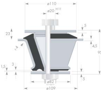
Art. Nr. 786026S1 NK 45°, NK 60° oder NK 70° Shore
