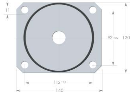
Art. Nr. 786030 NK 40°, NK 60° oder NK 70° Shore
