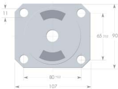
Art. Nr. 786026S3 NK 45°, NK 60° oder NK 70° Shore
