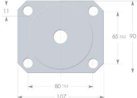
Art. Nr. 786026S1 NK 45°, NK 60° oder NK 70° Shore
