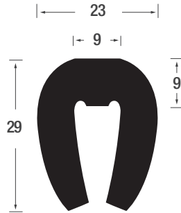
Art. Nr. U9/9 Material EPDM 60° Shore Farbe schwarz OR 20 m
