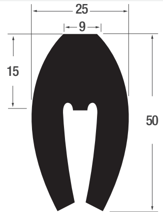
Art. Nr. U9/15 Material EPDM 60° Shore Farbe schwarz OR 20 m
