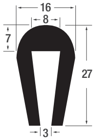
Art. Nr. W4713 Material EPDM Farbe schwarz OR 30 m
