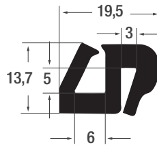
Art. Nr. D1013 Material EPDM Farbe schwarz OR 50 m
