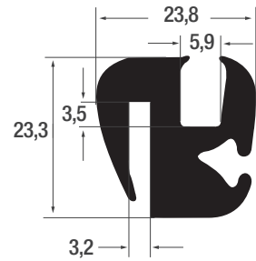
Art. Nr. B2144 Material EPDM Farbe schwarz OR 25 m
