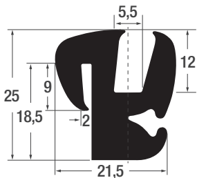
Art. Nr. B1117 Material EPDM Farbe schwarz OR 15 m
