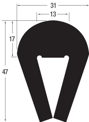
Art. Nr. U13/17 Material EPDM 60° Shore Farbe schwarz OR 20 m
