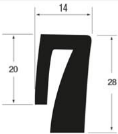
Silotürdichtprofil
