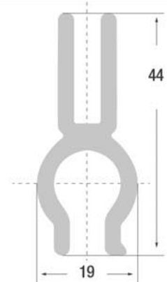
(Scharnier passend zu Profil P017)
